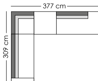
39: L 230 + 460 + 700 + R 213
