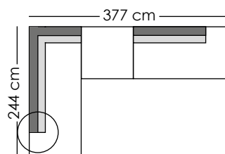
38: L 613 + 700 + R 213
